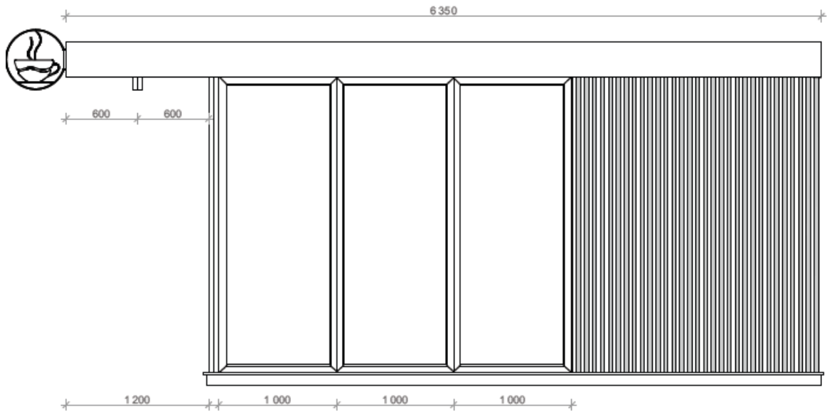
Рис. 45 Задний фасад
