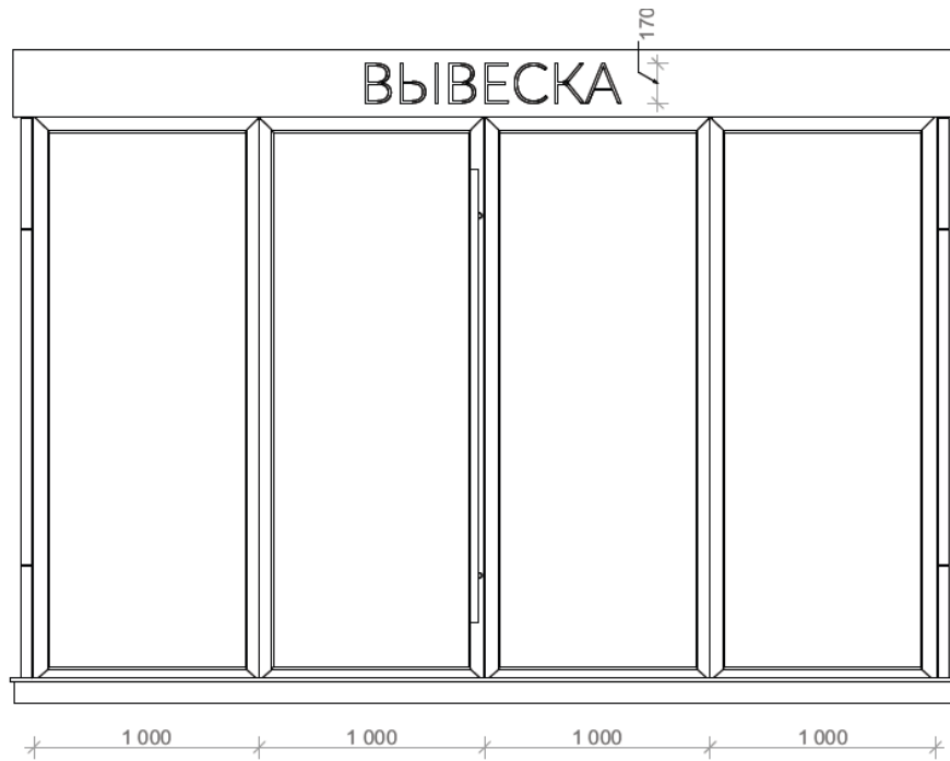
Рис. 33 Лицевой фасад
