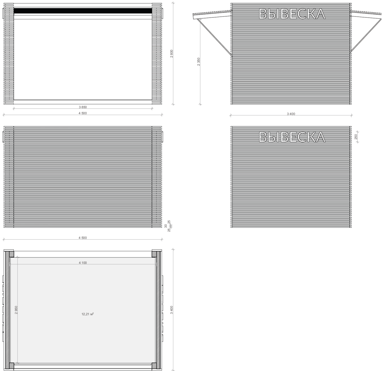
Рис. 58 Габаритные размеры
