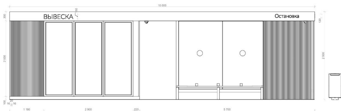
Рис. 51 Лицевой фасад
