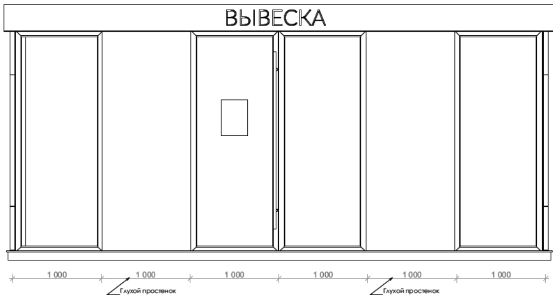
Рис. 38 Лицевой фасад
