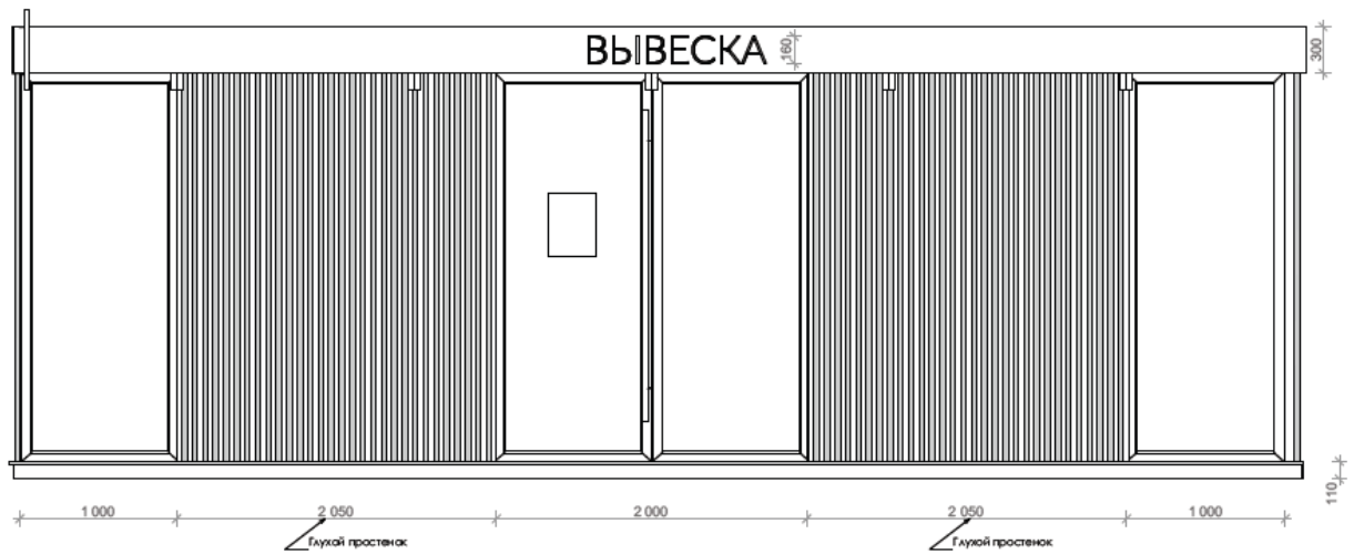
Рис. 44 Лицевой фасад
